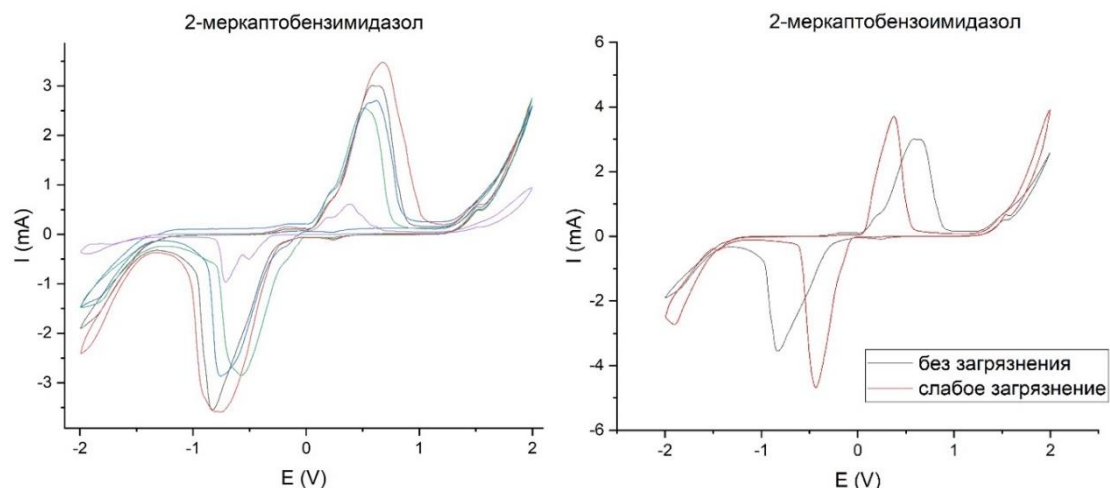
Рис. 3. Вольтамперограммы слабозагрязненной воды, содержащей 40 г/м 3 ингибитора 2-меркаптобензимидазол
